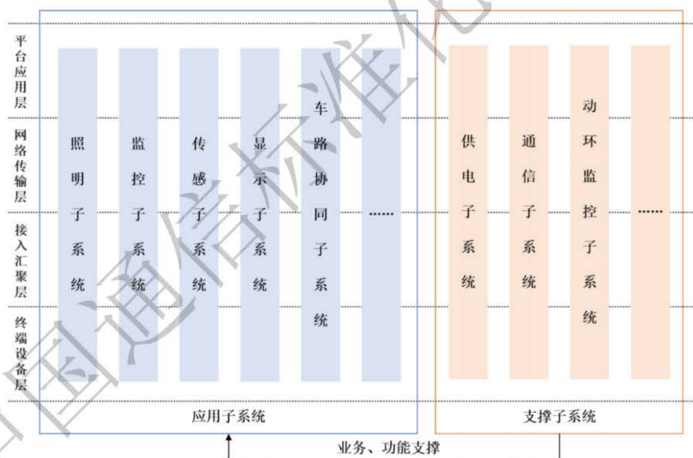
图 1-3 智慧杆塔系统架构（水平方向）示意图
