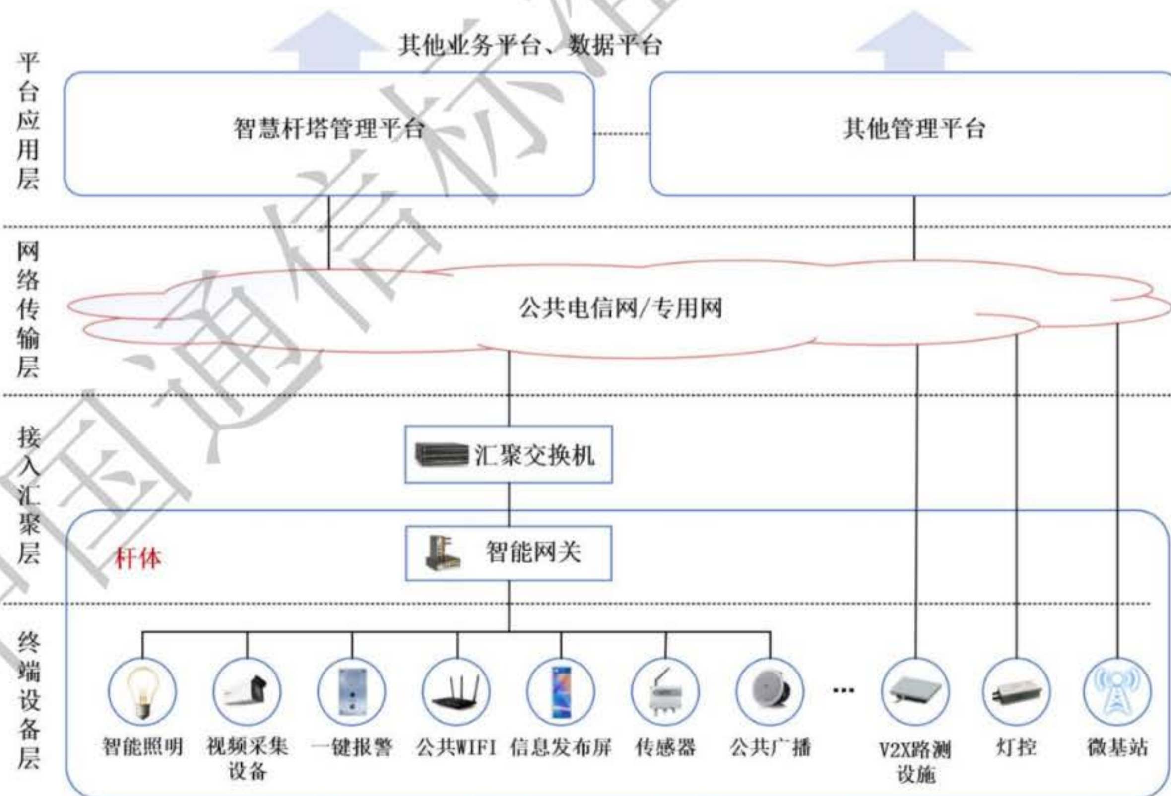
图 1-2 智慧杆塔系统架构（垂直方向）示意图
