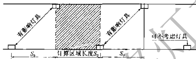
图 10-2 计算区域
