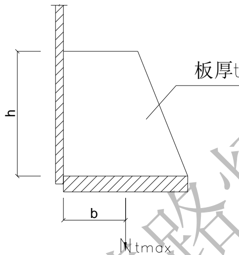
图B.2 肋板计算示意
