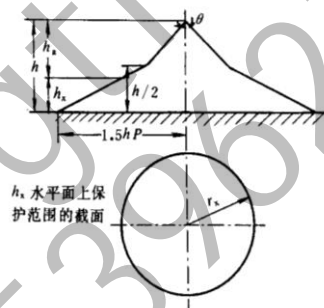
图 A.1 单支接闪针的保护范围
