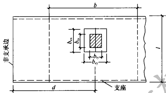
图 C.0.5-1 简支板上局部荷载的有效分布宽度 (荷载作用面的长边平行于板跨)
