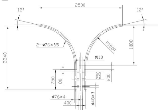
图 3.3.3-10 灯臂尺寸
