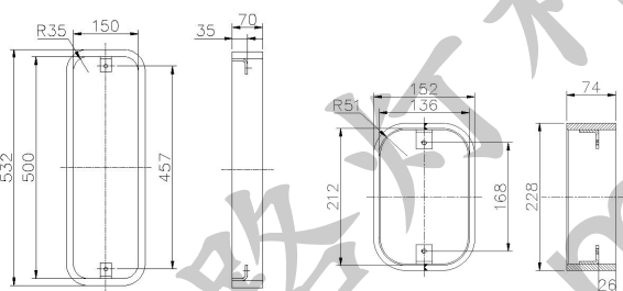
图 4.2.2-1 主检修门
