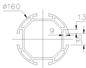
图 4.2.4 副杆截面
