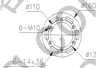
图 3.3.3-5 法兰 6
