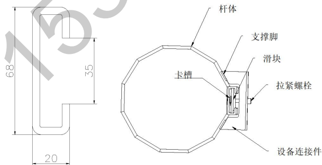
图 4.2.1 卡槽截面及设备连接件连接示意
