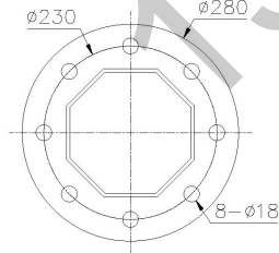
图 3.3.3-9 法兰 10
