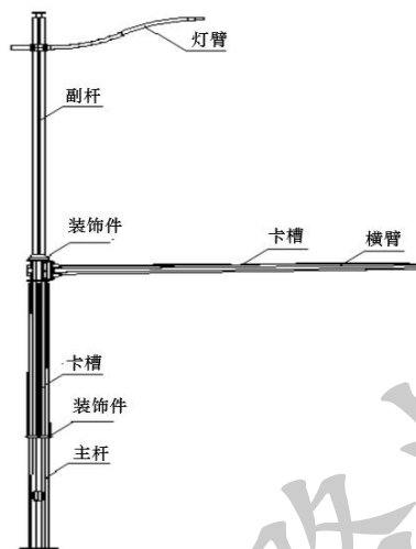
图 3-2 多功能智慧灯杆基本组成示意图
