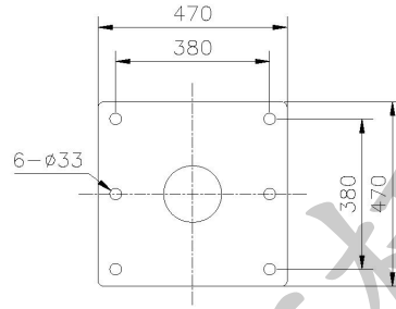
图 3.3.3-2 法兰 2
