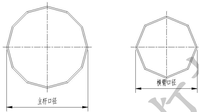
图 3.3.1 主杆及横臂口径
