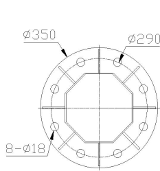
图 3.3.3-3 法兰 3
