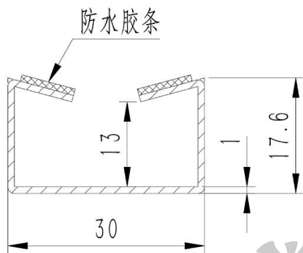
图 3.4.2.3-1 压线条尺寸图
