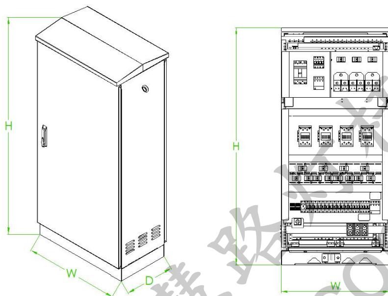
图9.2.4.1-1 综合配电箱结构、尺寸示意图
