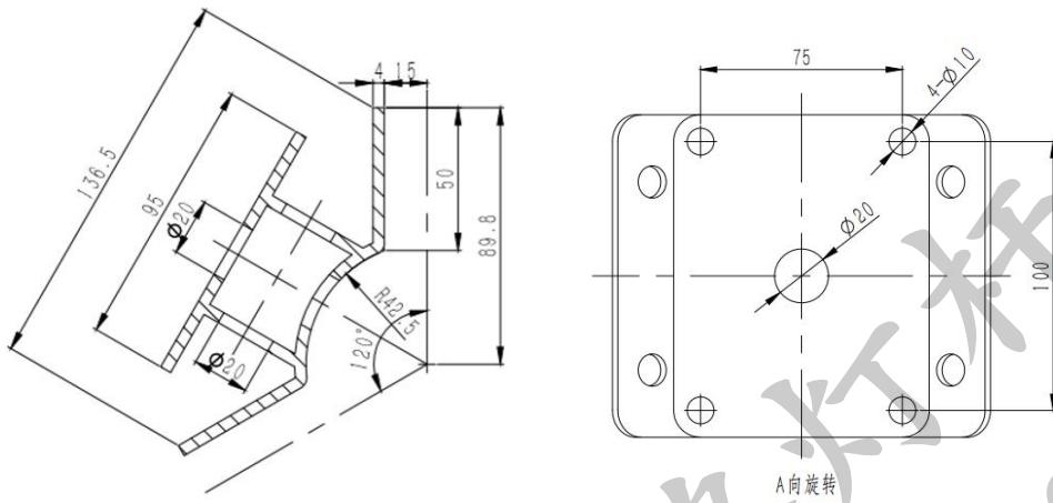
图 3.4.2.2-1 转接环尺寸
