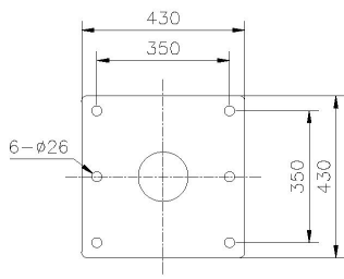
图 3.3.3-1 法兰 1
