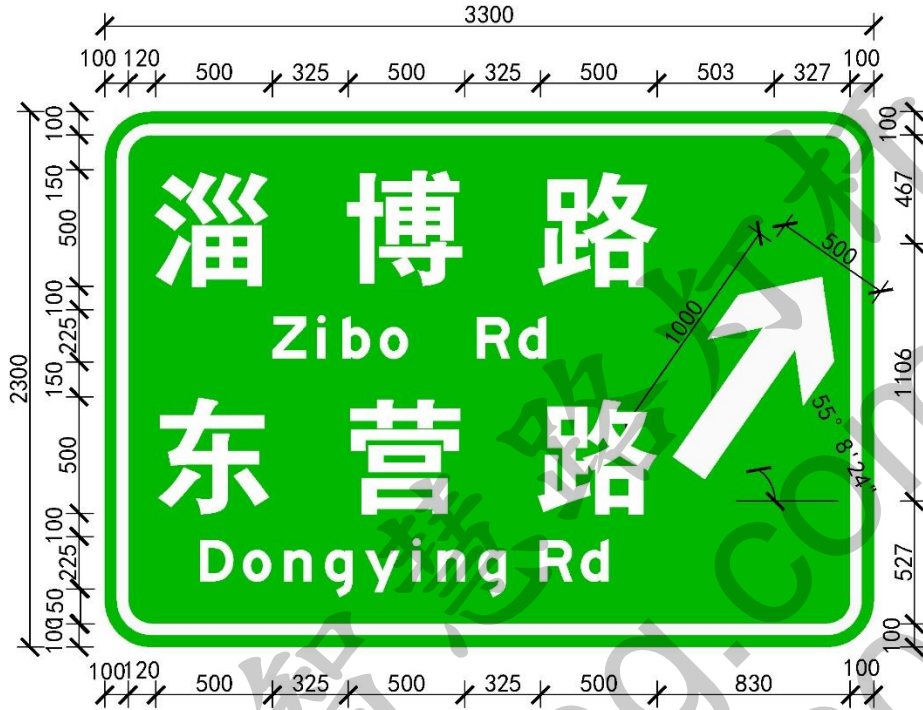
图F.3 快速路出口预告标志
