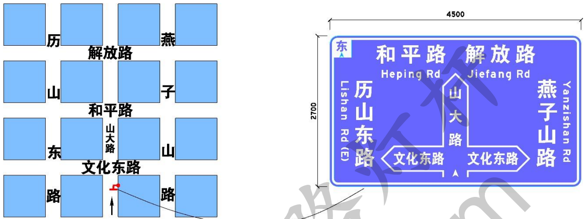
图F.7 交叉口告知标志版面信息含义
